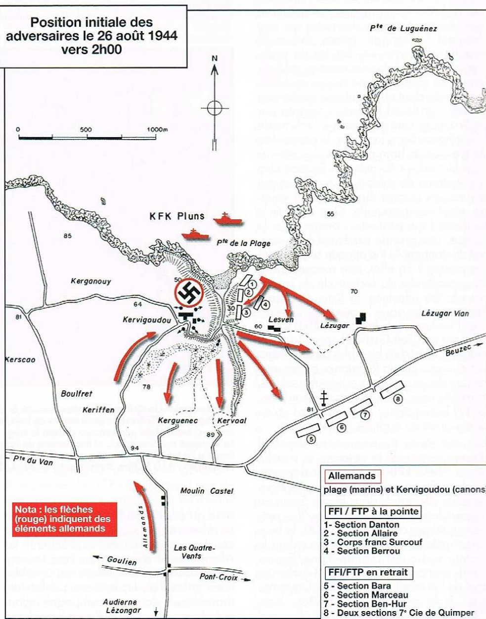
Carte du secteur de Lesven-Kervigoudou indiquant les positions des FFI/FTP dans la nuit du 25 au 26 août 1944 et les mouvements allemands (flèches) dans la matinée du 26.
